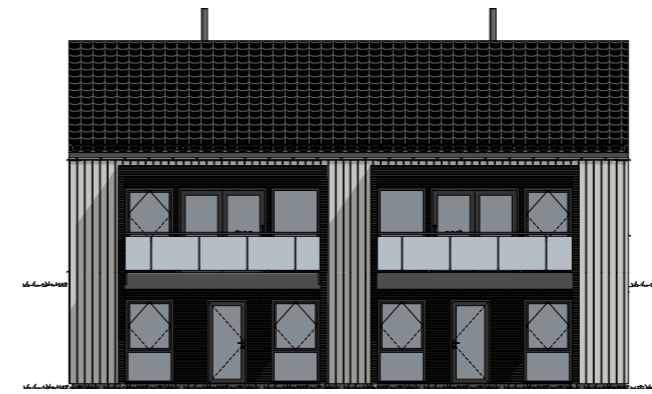
FASADE SØR
