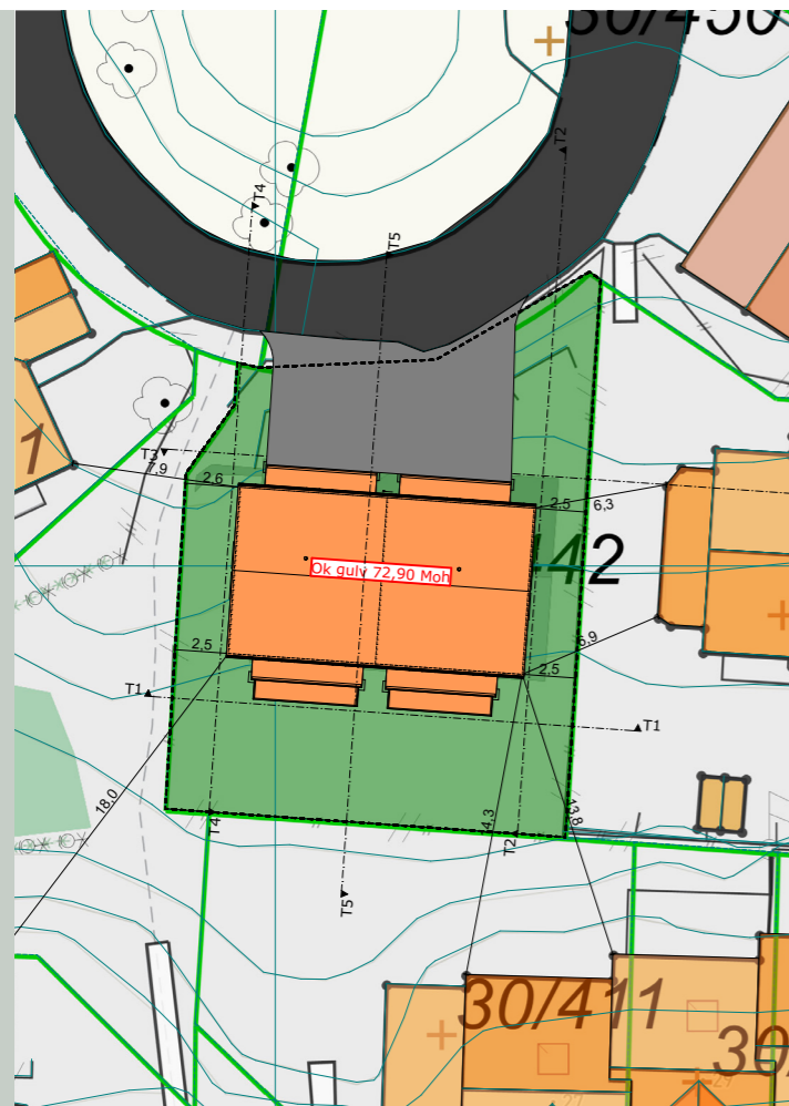
SITUASJONSPLAN
